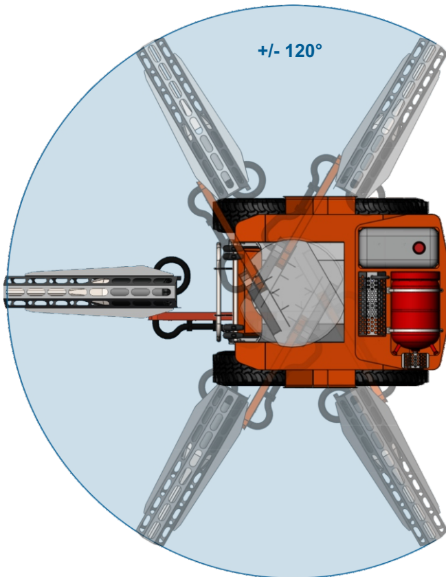
Drehwinkel der Dampfkanone +/- 120° einstellbar.
